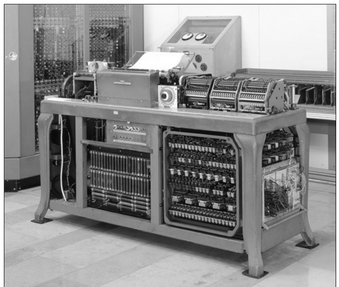
Dehomag Tabulator D11
